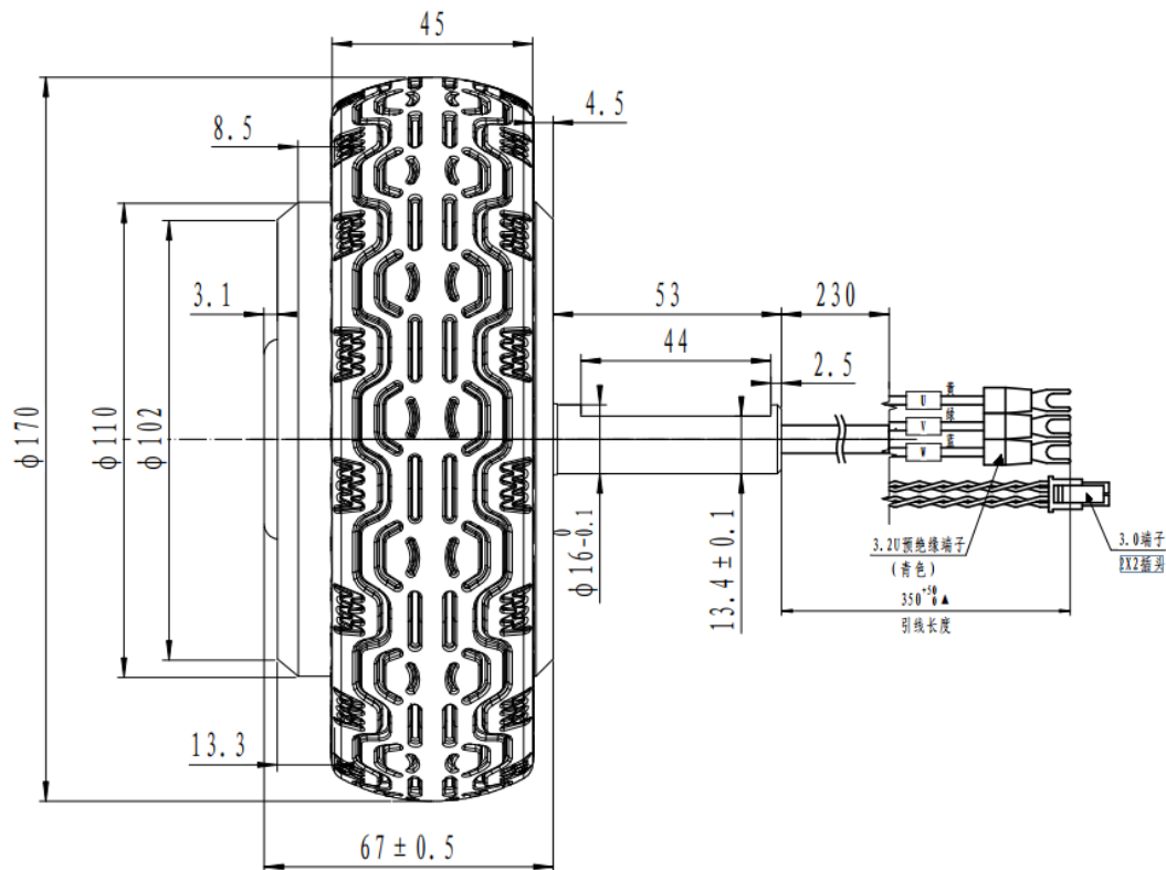
图 3.1.2 6.5 寸轮毂电机安装尺寸
