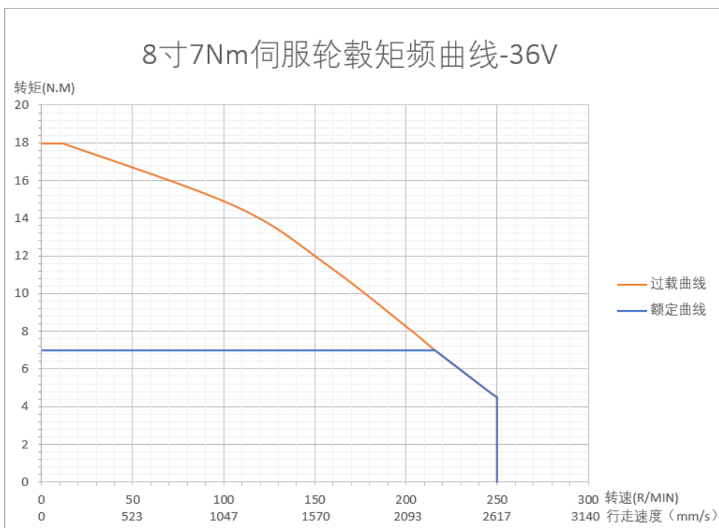
图 2.1.3-1 6.5 寸 7Nm 轮毂电机特性曲线
