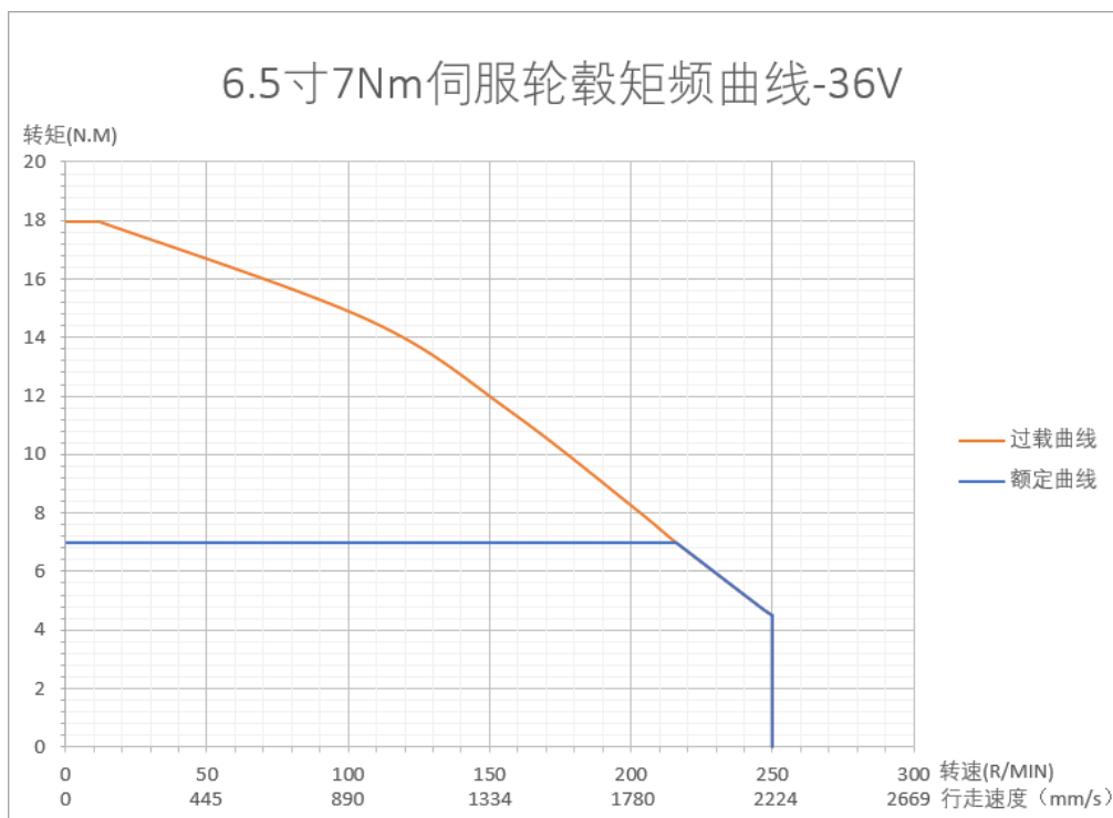
图 2.1.2-1 6.5 寸 7Nm 轮毂电机特性曲线
