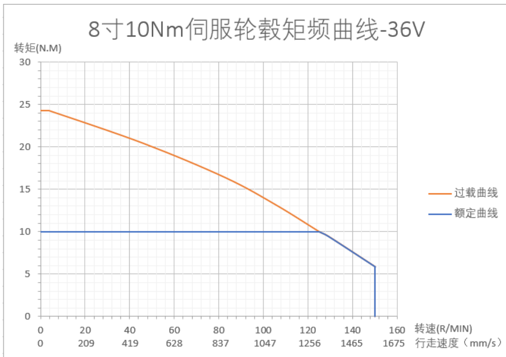
图 2.1.4-1 8 寸 10Nm 轮毂电机特性曲线
