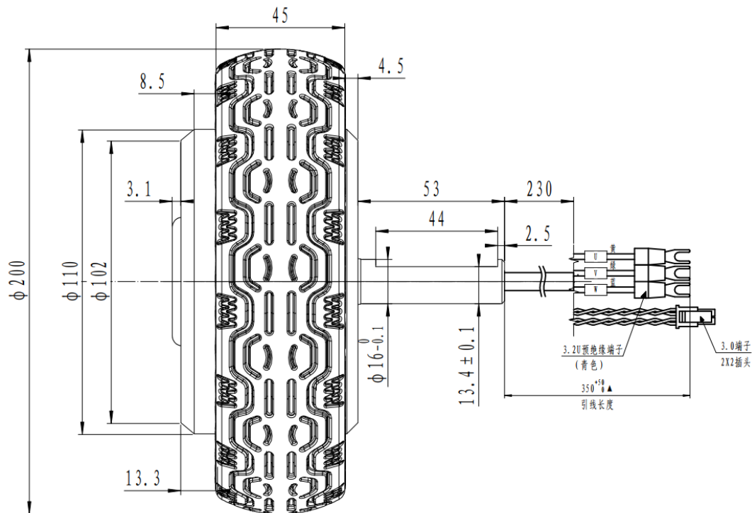
图 3.1-3 8 寸 7Nm 轮毂电机安装尺寸
