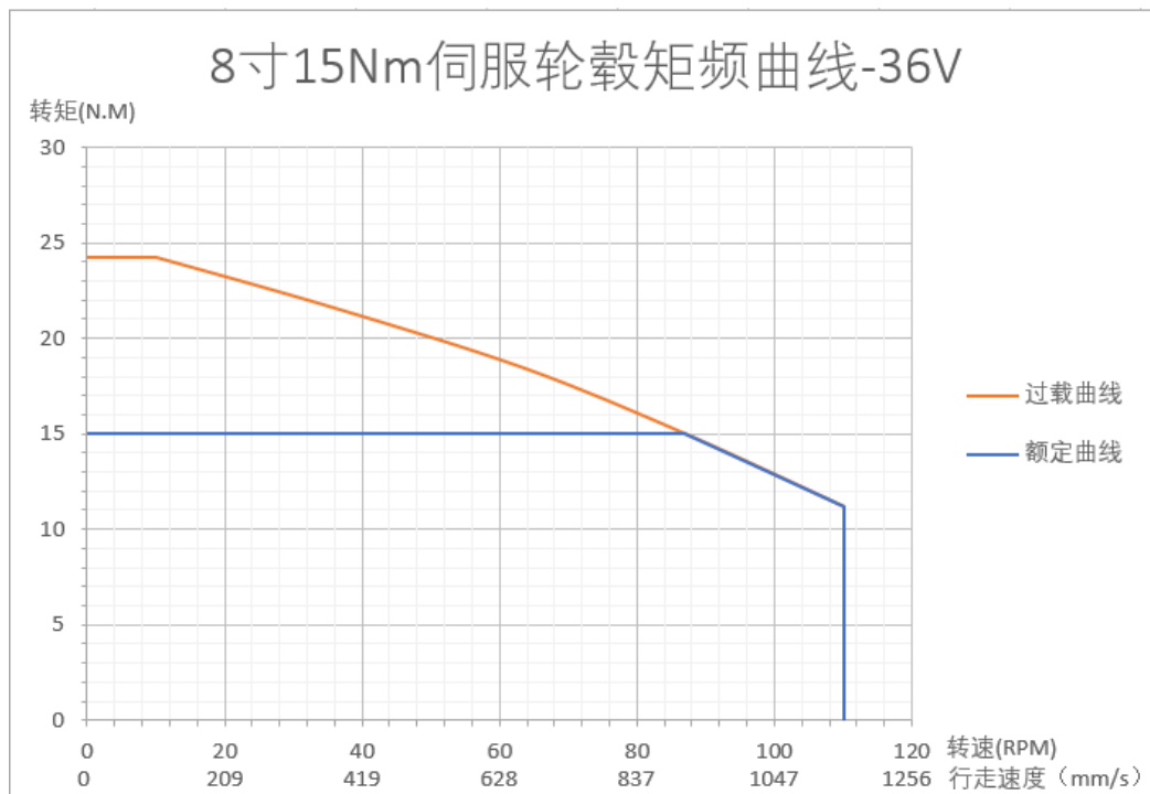
图 2.1.5-1 8 寸 15Nm 轮毂电机特性曲线
