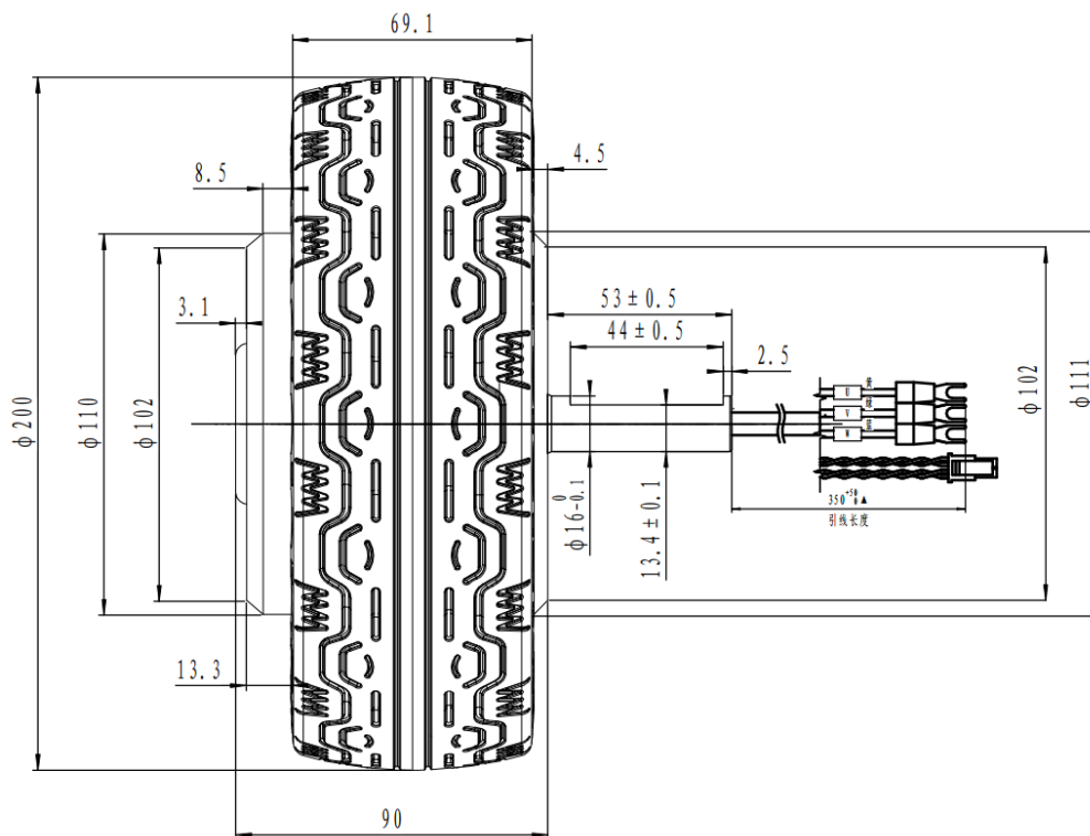
图 3.1-5 8 寸 15Nm 轮毂电机安装尺寸
