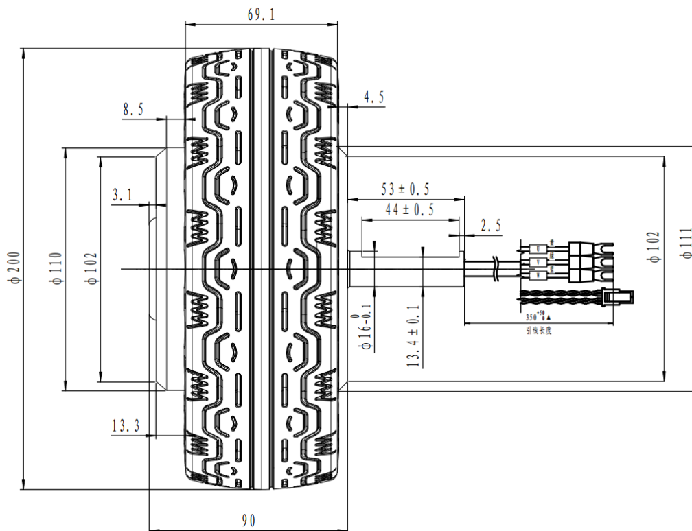
图 3.1-4 8 寸 10Nm 轮毂电机安装尺寸
